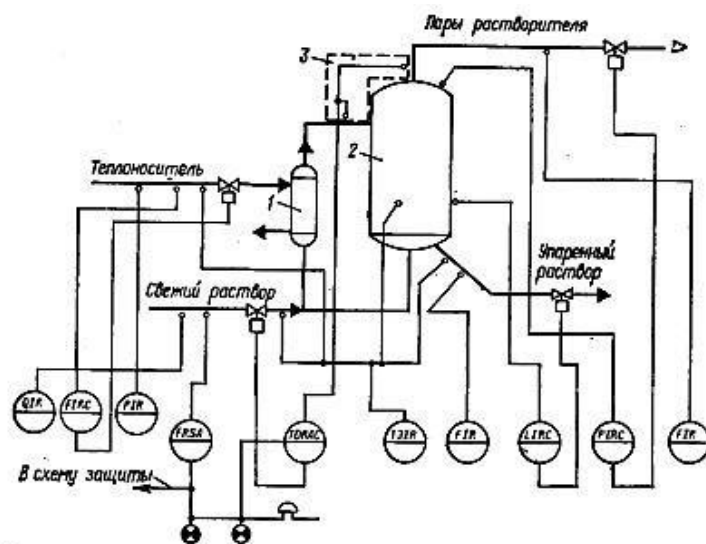
Рисунок 1 - Типовая схема автоматизации процесса выпаривания:
